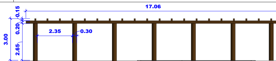
4 Det. Pergolado 1 : 100
